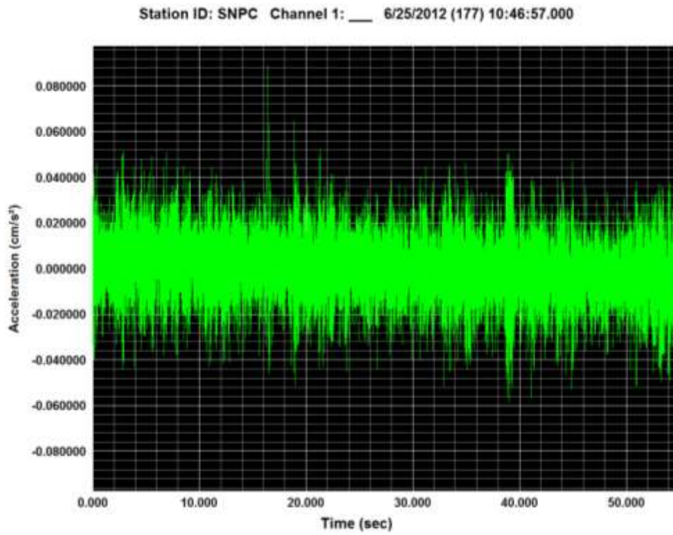
Figura 7: Traçado da componente X, diametral, do registo CY005 (local A1).
